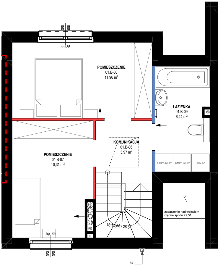
RZUT 1 PIĘTRA
